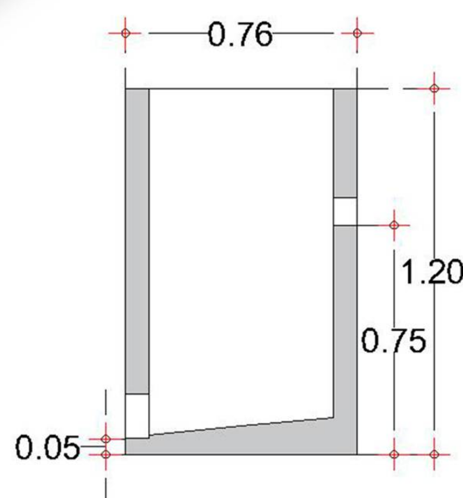
VISTA EN CORTE
