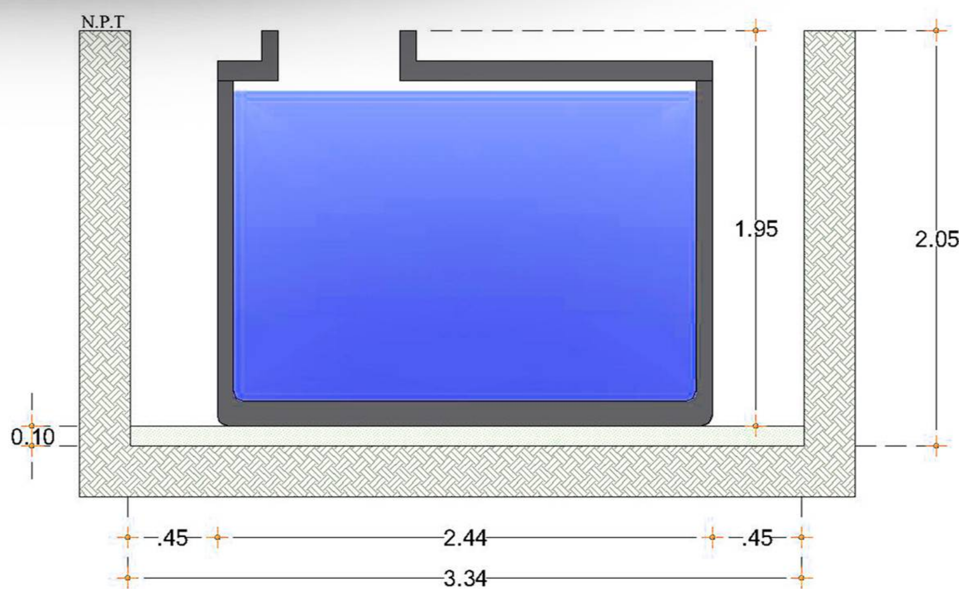
VISTA EN CORTE
