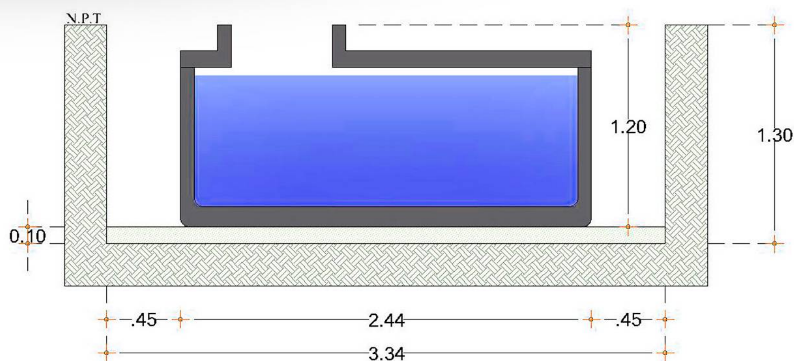
VISTA EN CORTE
